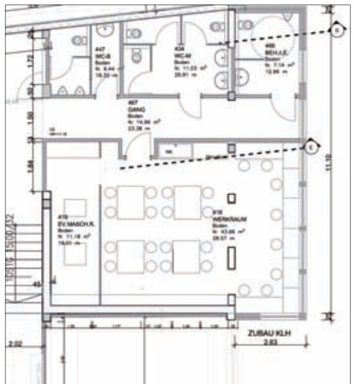
Grundriss – geplanter neuer Werkraum der Volksschule.
