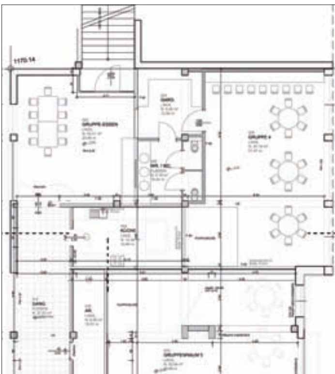
Grundriss – geplante Kindergartenerweiterung.
